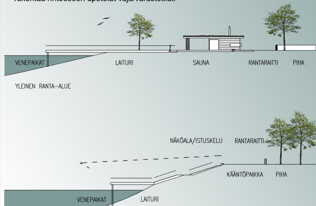
LEIKKAUKSET 1:500
